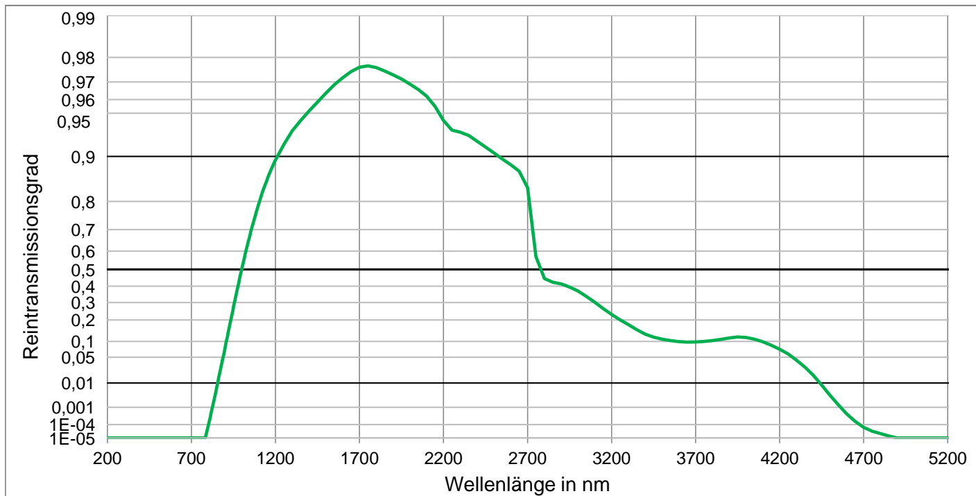
Reintransmissionsgrad \tau_i bei der Referenzdicke
