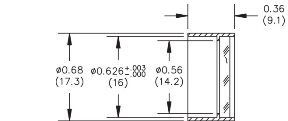
A08087 Input Lens Diffuser (Opal)
